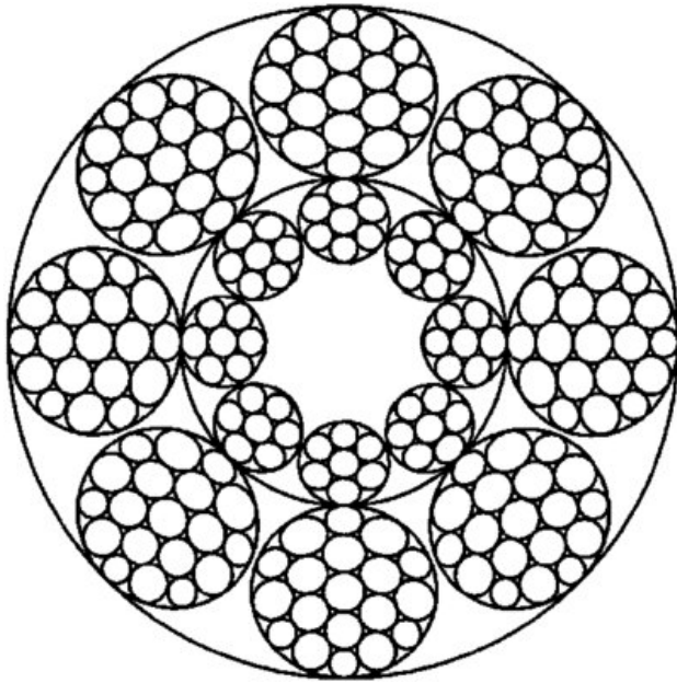
Aufzugseil
