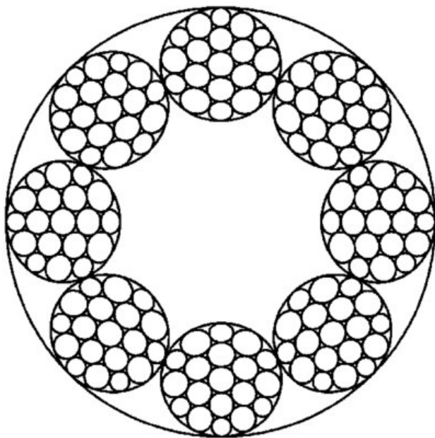
Aufzugseil
